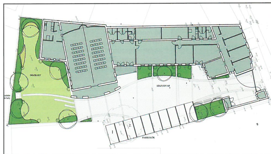
Az ügyfélszolgálati irodák és a házasságkötő terem alaprajza
